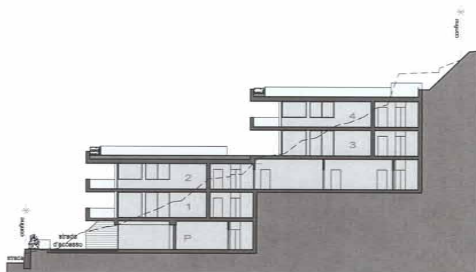
Sezione
